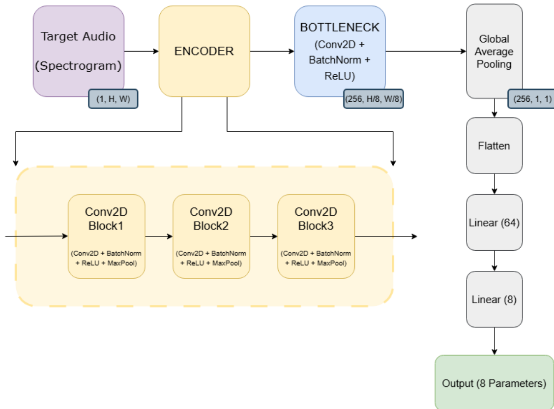
Figura 3.1: Representación de la estructura interna de CNNRegressorSimple.
